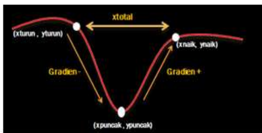
Gambar 7. Input NN
