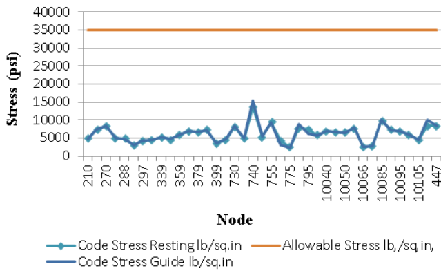
Gambar 3. Hasil Tegangan Hydrotest pada pipa 24 inch
