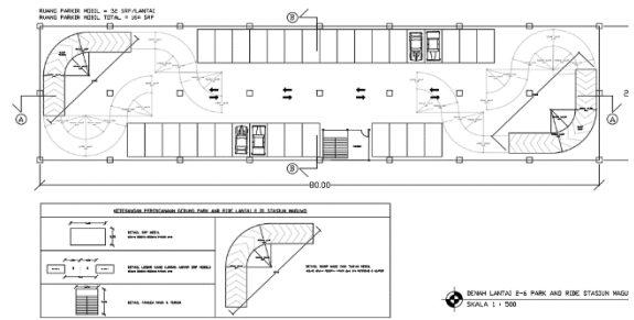
Gambar 5. Layout Gedung Park and Ride Stasiun Maguwo Lantai 2-6.
