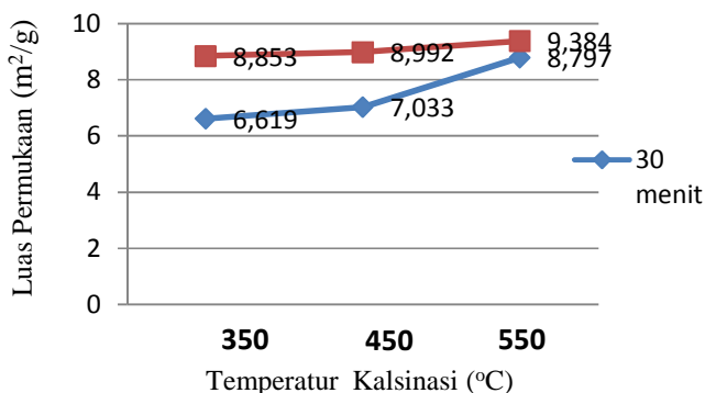
Gambar 5. Grafik hubungan temperatur kalsinasi dan waktu tahan terhadap luas permukaan aktif Titanium Dioksida (TiO 2 )
