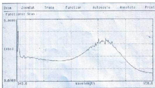
Gambar 1. Grafik absorbansi ekstrak buah naga merah
