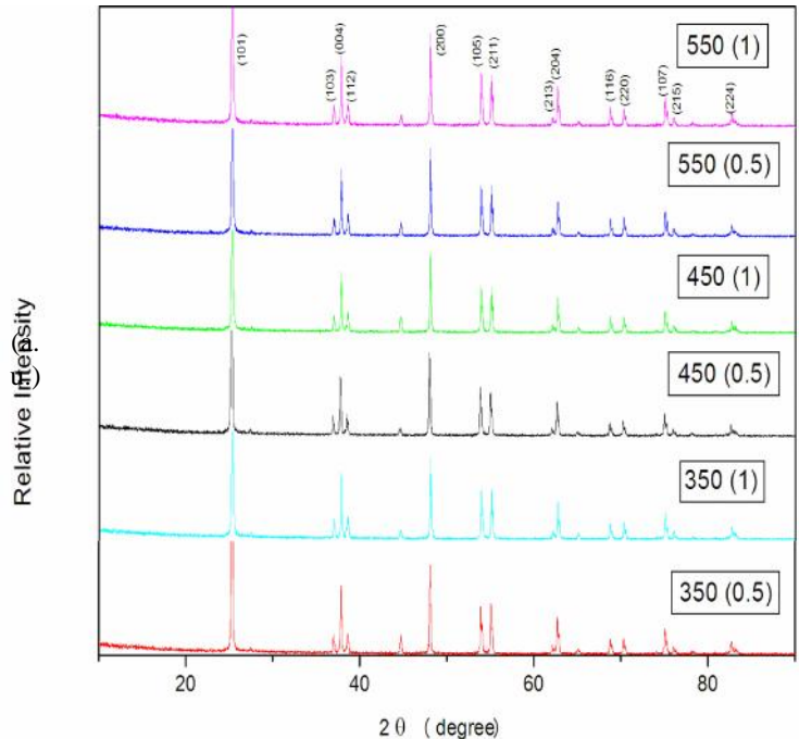
Gambar 2. Pola XRD pada lapisan Titanium Dioksida (TiO 2 ) yang telah dikalsinasi dengan variasi temperatur (a-b) 350°C, (c-d) 450°C, (e-f) 550°C dan waktu tahan 30 menit dan 60 menit
