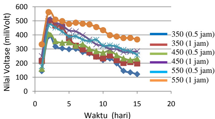
Gambar 6. Grafik hubungan variasi temperatur dan waktu tahan terhadap DSSC buah naga merah
