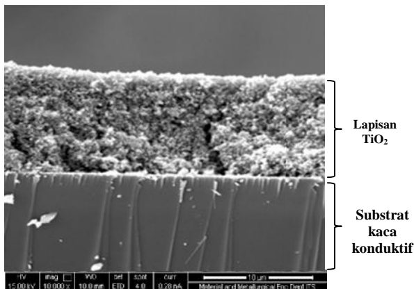
Gambar 3. Hasil Foto SEM cross section Titanium Dioksida (TiO 2 ) pada temperatur kalsinasi 450°C dengan perbesaran 10.000x
