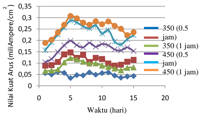
Gambar 7. Grafik hubungan variasi temperatur dan waktu tahan terhadap kuat arus DSSC buah naga
