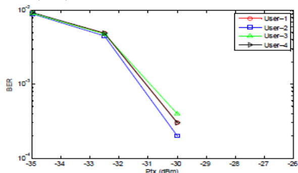
Gambar 13 Grafik BER saat Pengiriman 4 User Hadamard 16 bersamaan
