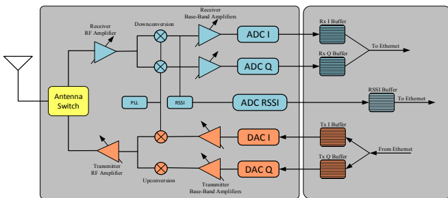
Gambar 5 Arsitektur WARPLab [4]
