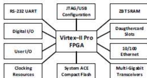
Gambar 3 Arsitektur hardware WARP [3]
