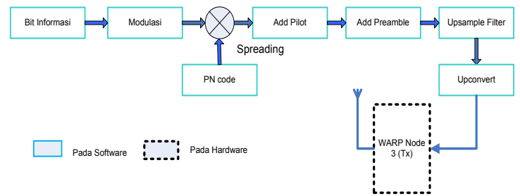
Gambar 6 Blok desain implementasi sistem transmitter
